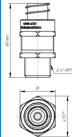
ВКВ-G3/4-M
