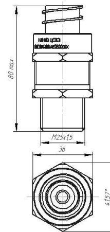
ВКВ-M25-M
