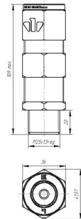
ВКВ-M25-Б
