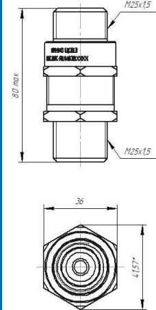
ВКВ-M25- M25-T
