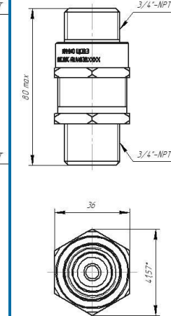
ВКВ-G3/4- G3/4-T
