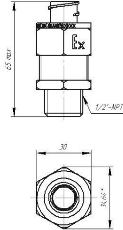
ВКВ-G1/2-M
