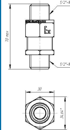
ВКВ-G1/2- G1/2-T
