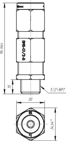
ВКВ-G1/2-Б
