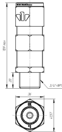
ВКВ-G3/4-Б
